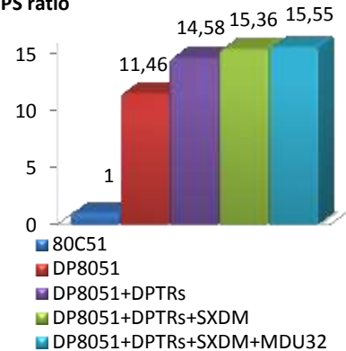
VAX MIPS ratio
